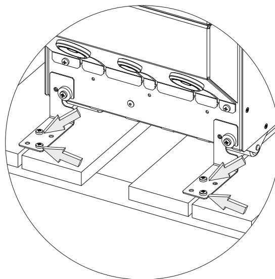
VISTA RETRO
